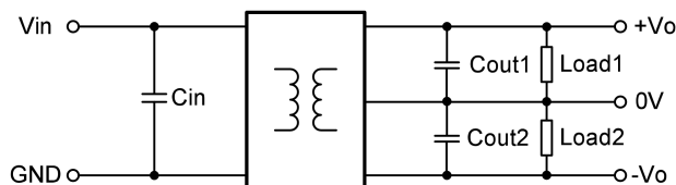
图 1 双路应用电路图
