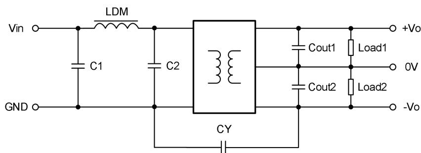
图 2 EMC 推荐电路图
