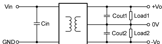
图 1 应用电路图
