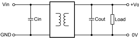
图 1 应用电路图
