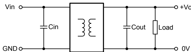
图 1 应用电路图
