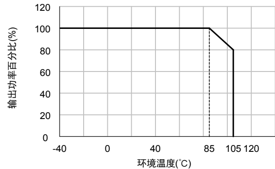
环境温度降额曲线图
