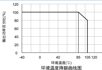
环境温度降额曲线图
