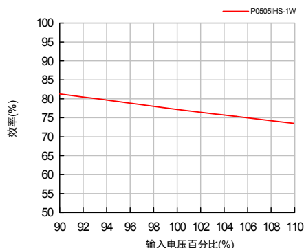
效率与输入电压关系曲线图 (满载)
