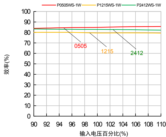
效率与输入电压关系曲线图 (满载)
