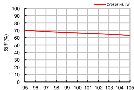
效率与输入电压关系曲线图(满载)
